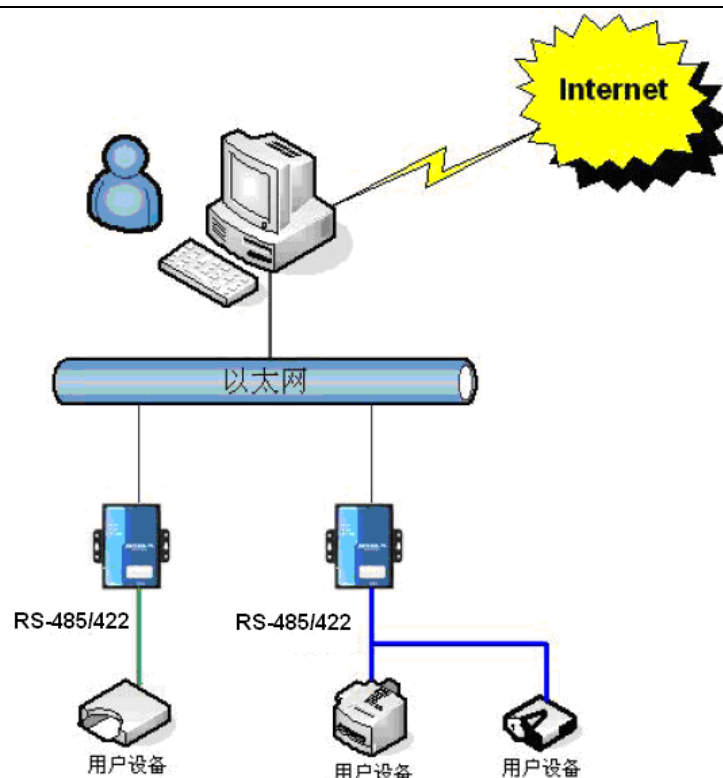
图 2 连接示意图
