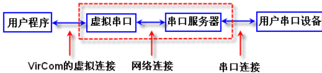
图 11 虚拟串口的作用
