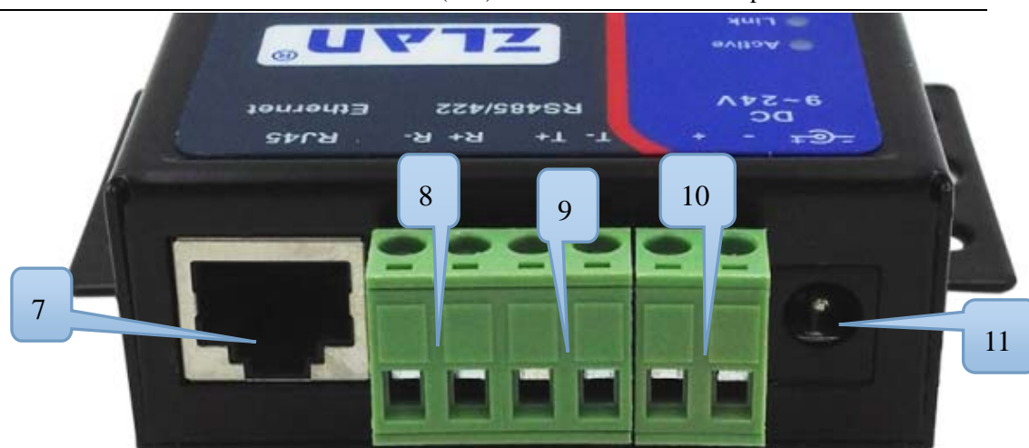
图 5 网口和 485 接口
