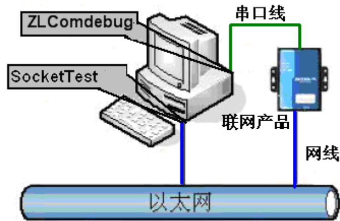
图 8 透传通信示意图
