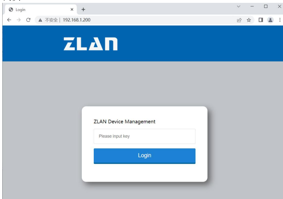
图 24 Web 登录页
