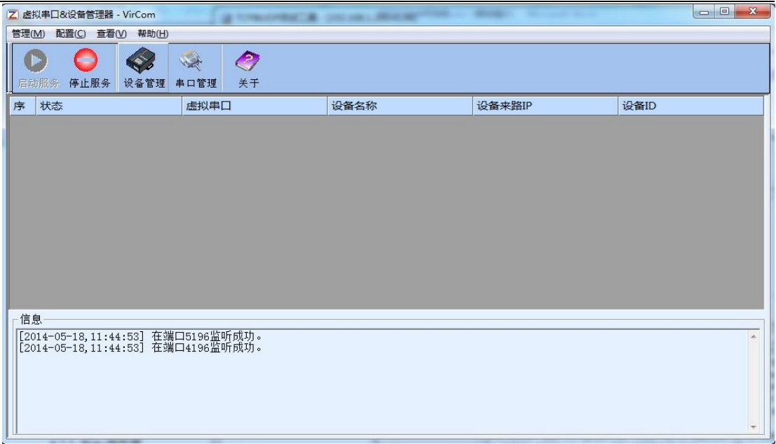
图 12 ZLVircom 主界面
