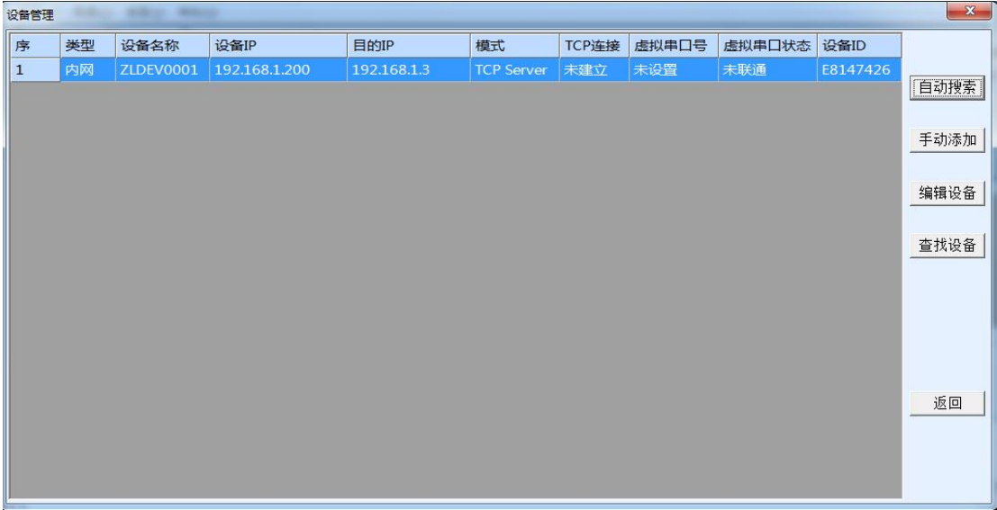
图 13 设备列表
