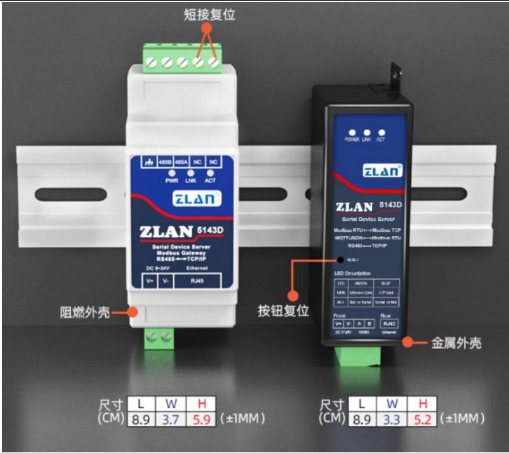
图 10 白色款和黑色金属款对比
