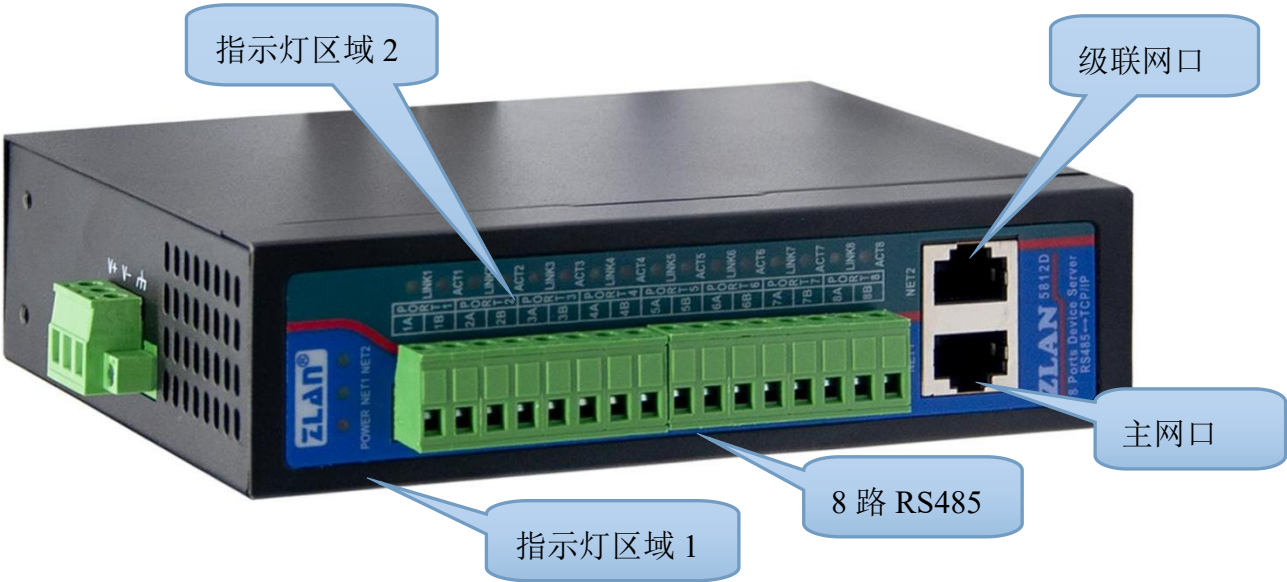
图 3 正视图
