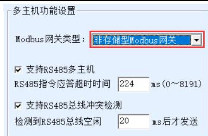
图 43 新版 zlvircom 的设置
