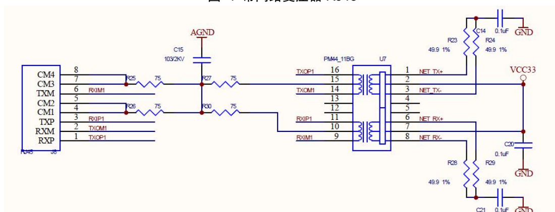
图 5 RJ45 和网络变压器分开方式
