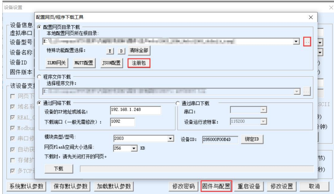
图 48 下载注册包
