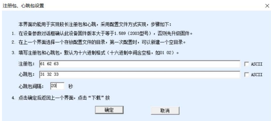
图 49 配置注册包
