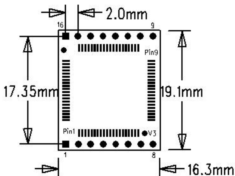
图 3 2007S 引脚图
