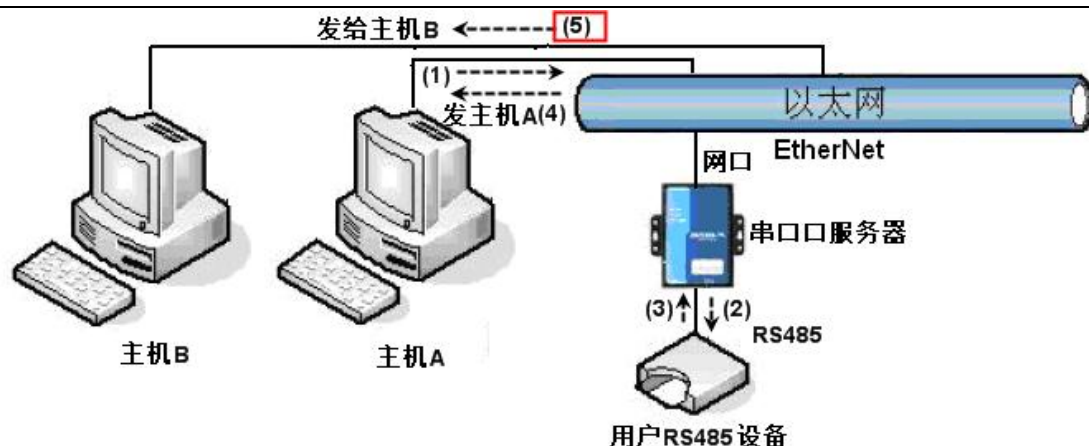
图 39 多主机功能演示
