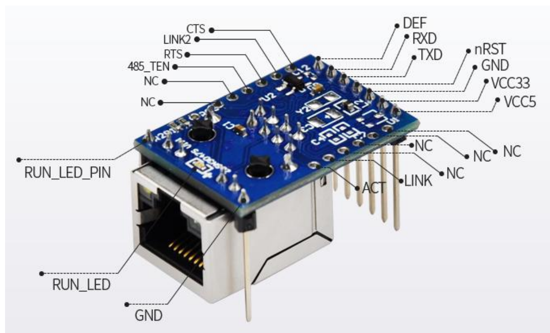
图 5 ZLSN3007S 引脚图
