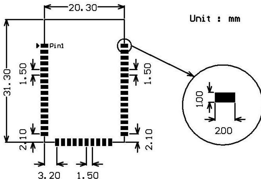
图 59 ZLSN7046T 封装尺寸
