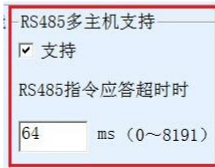
图 39 RS485 多主机支持
